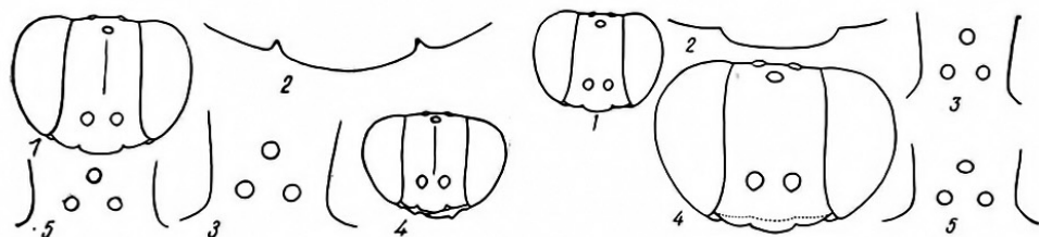
Рис. 1. Miscophus rasilis Kazenas, sp. n.: 1 — лицо спереди; 2 — передний край срединной лопасти наличника; 3 — темя сверху; 4 — голова спереди; 5 — темя сверху; 1—3 — самка; 4, 5 — самец.
